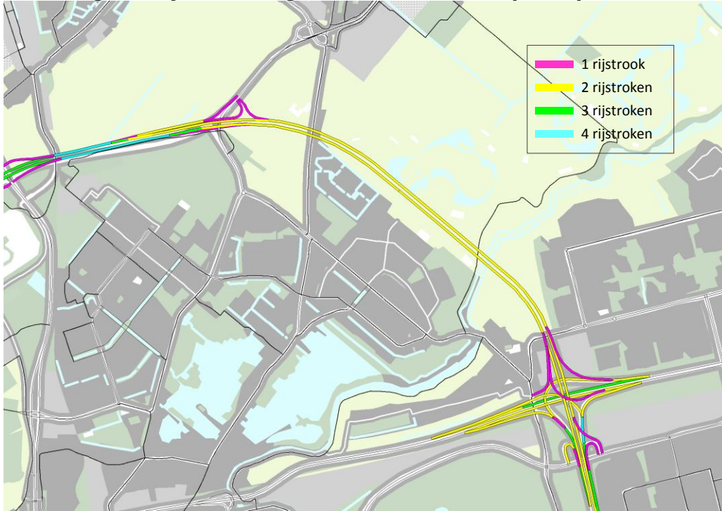
Afbeelding 3.2. Rijstrookconfiguratie A16 Rotterdam (deel 2)
