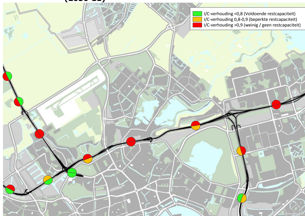
Afbeelding 4.5. Benutting hoofdwegennet avondspits in referentiesituatie (2030 GE)
