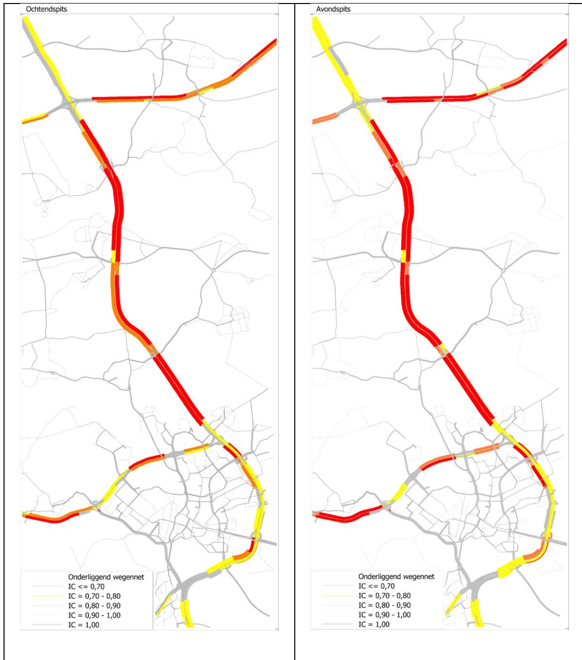
Afbeelding 5.8 Verhouding tussen intensiteit en capaciteit op het hoofdwegennet in de ochtend- en avondspits in Referentie 2040 Hoog
