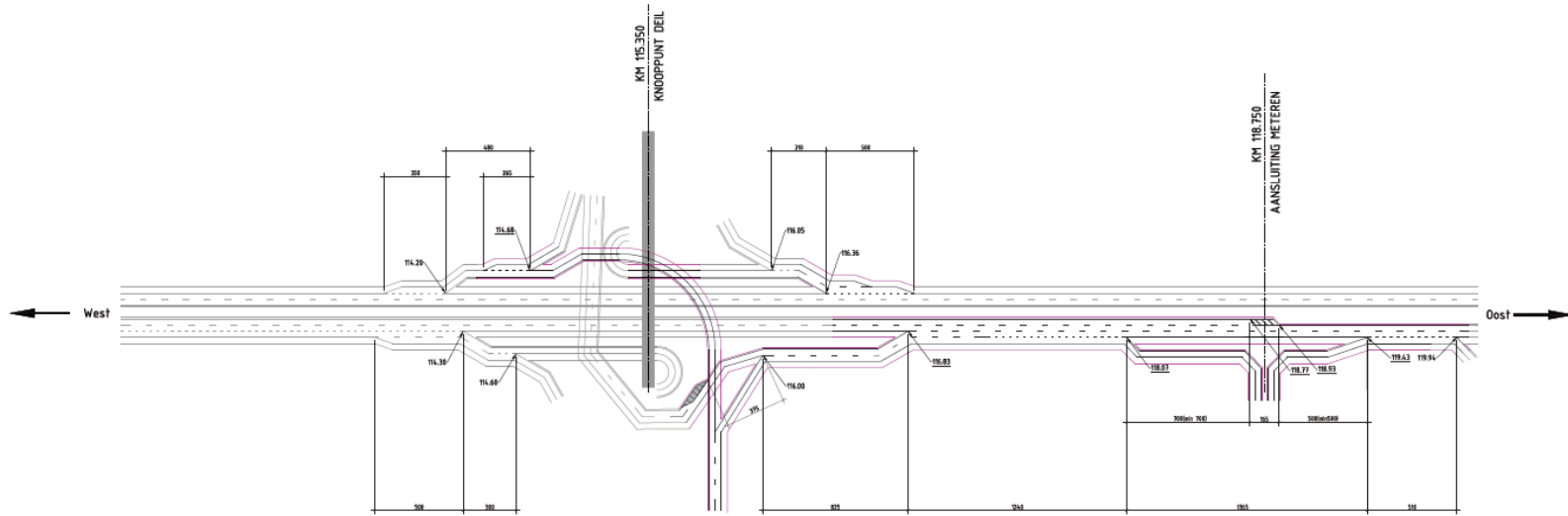
Afbeelding I.3 Rijstrokenschema Deil alternatief B (knelpunt 1: variant 3, knelpunt 2: variant 2, knelpunt 4: variant 2)
