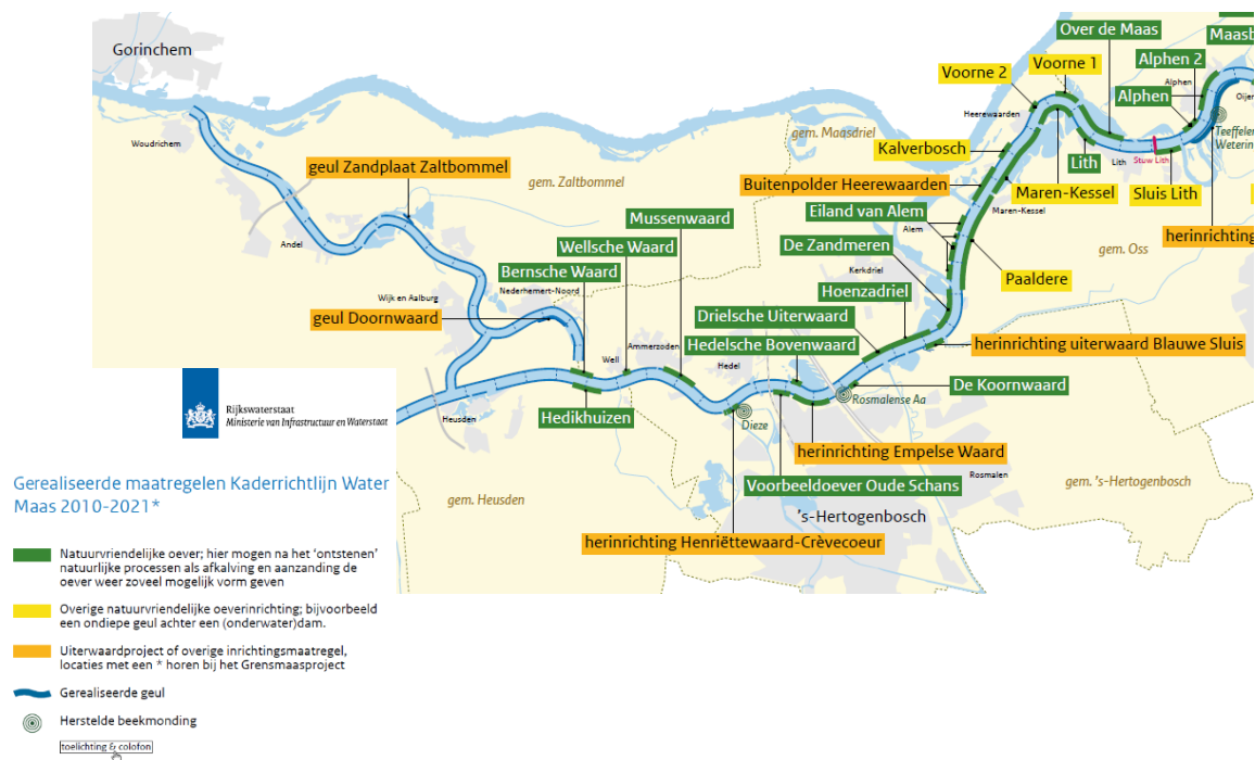
Figuur 4.1 Overzichtskaart gerealiseerde maatregelen in de Beneden Maas tussen 2010 en 2021, inclusief ecologische herstelmaatregelen van vóór de start van de KRW (RWS, Ministerie IenW, 2023a)
