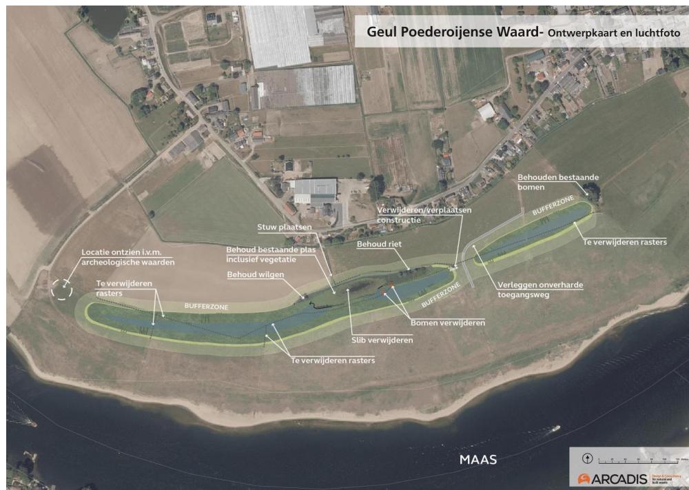
Figuur 5.3 Ontwerpkaart Geul Poederijense Waard (MIRT3) (Arcadis, 2023)
