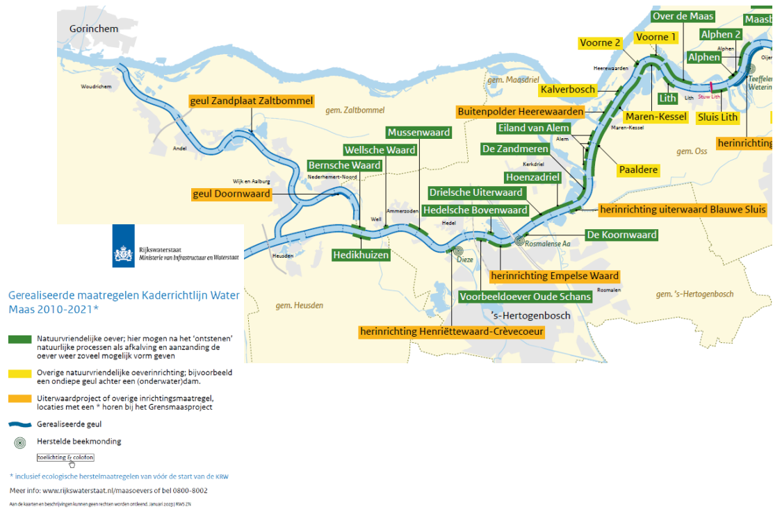
Figuur 4.1 Overzichtskaart gerealiseerde maatregelen in de Beneden Maas tussen 2010 en 2021, inclusief ecologische herstelmaatregelen van vóór de start van de KRW (RWS, Ministerie IenW, 2023a)
