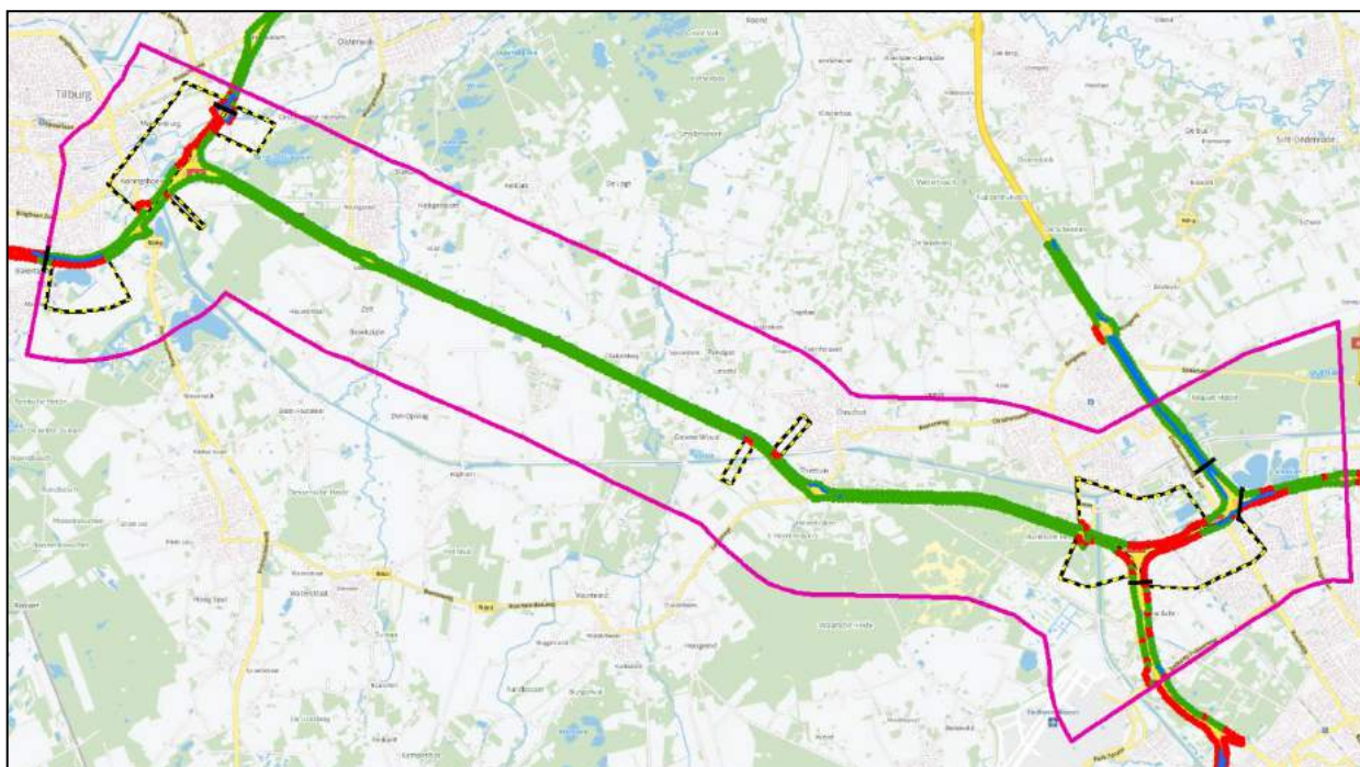
Figuur 5-5 Toetsing projectsituatie aan geldende geluidproductieplafonds voor de autonome situatie
