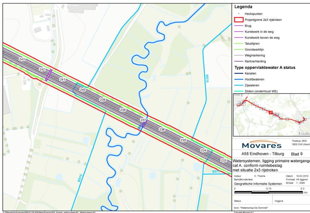
Figuur 6-1 Voorbeeld kruising primaire watergang
