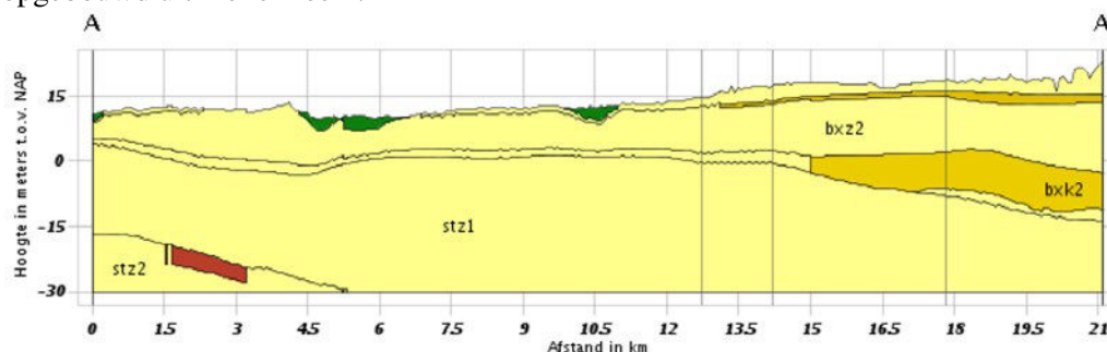
Figuur 7-1 Bodemopbouw langs tracé
