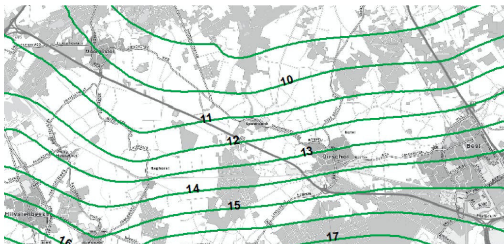
Figuur 7-2 Isohypsens grondwater (bron DINO - map, opname 28-04-1995)
