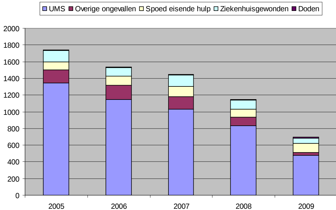
Afbeelding 6.2: Ontwikkeling slachtofferongevallen op het OWN binnen het invloedsgebied.
