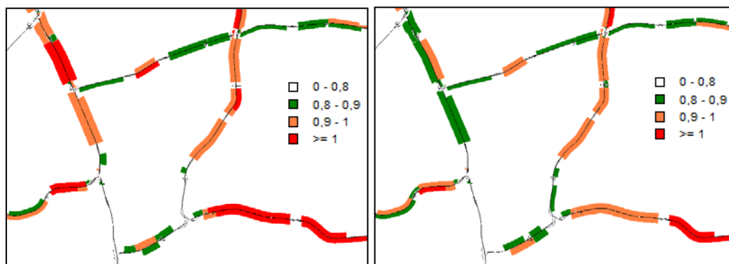
Figuur 6: IC verhouding ochtendspits (links) en avondspits (rechts) 2x2 met spitsstroken (GE)
