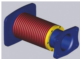
Figuur 5: Voorbeeld Crashbuffer (4 per ketelwagen).
