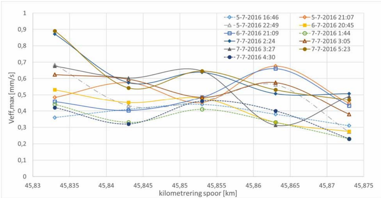
Figuur 19 Goederentreinen uit overweg meting Orthen (doorgetrokken streep treinen westelijk spoor, stippellijn oostelijk spoor)
