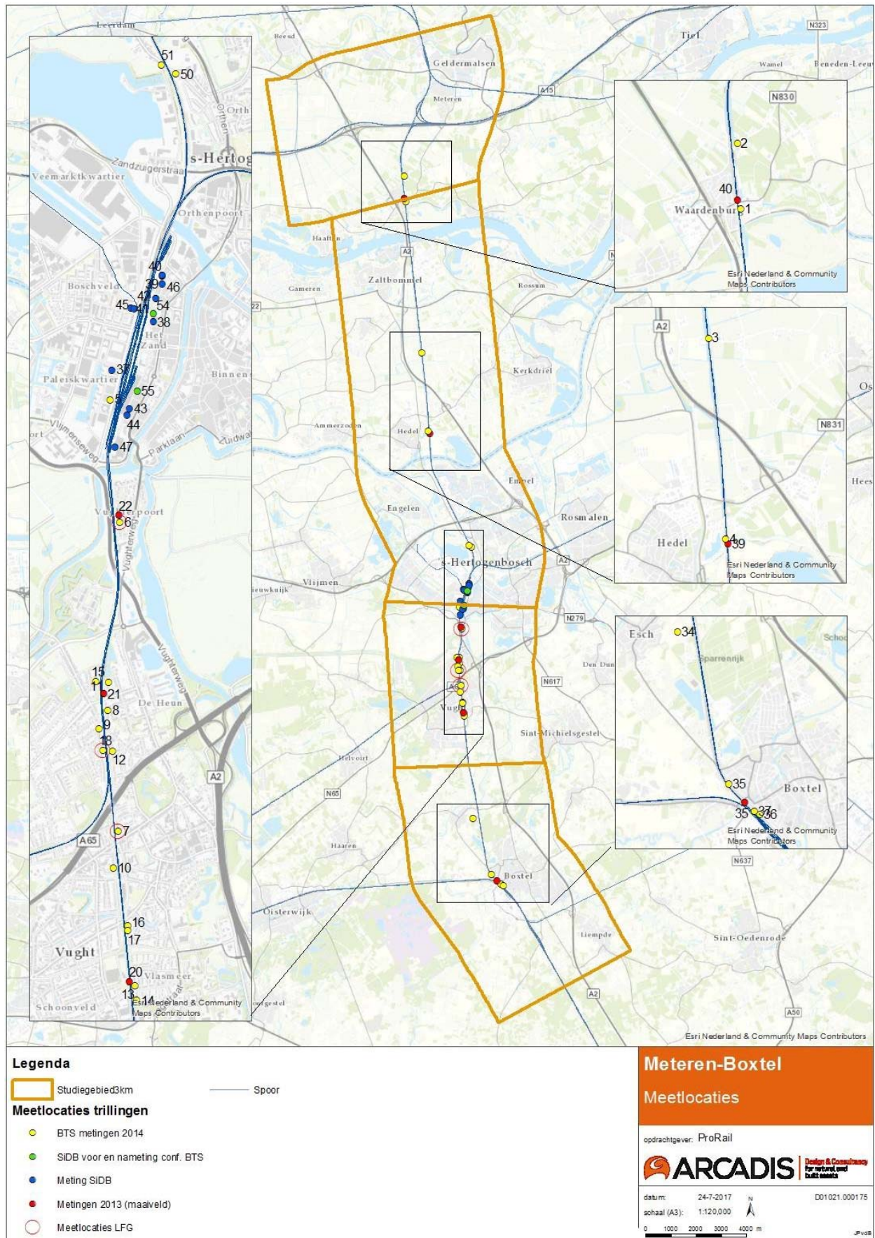
Figuur 15 Overzicht meetlocaties trillingen
