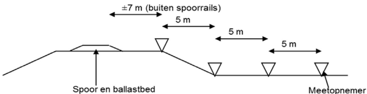
Figuur 16 Meetopstelling ten behoeve van demping grond (meetraai)
