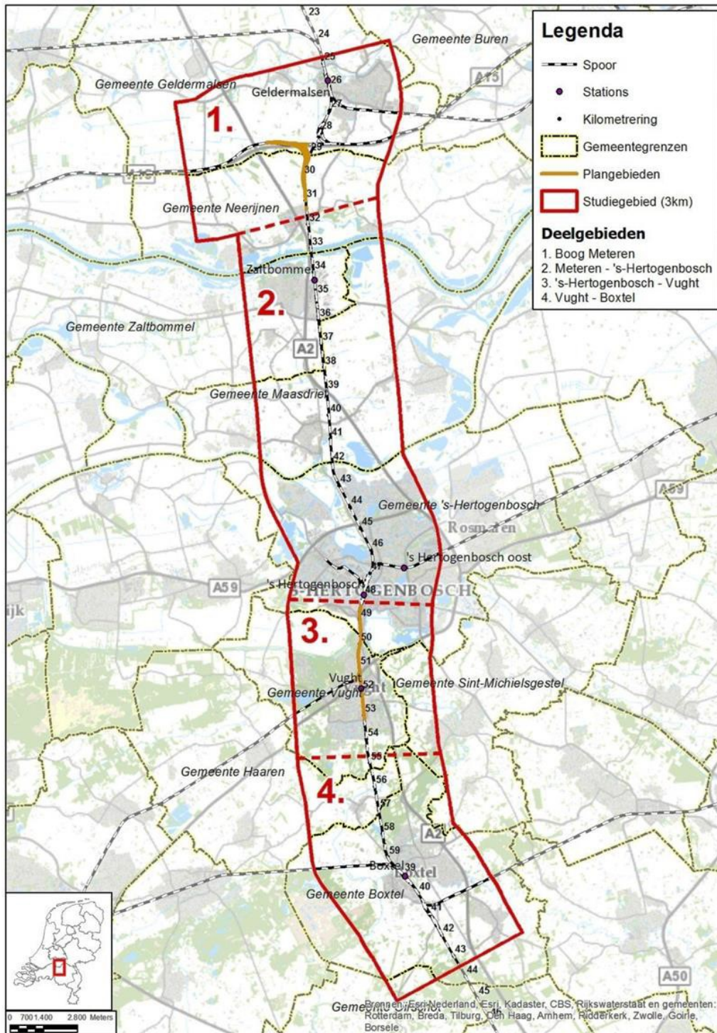
Figuur 4: Studiegebied Meteren - Boxtel: Plangebieden en deelgebieden
