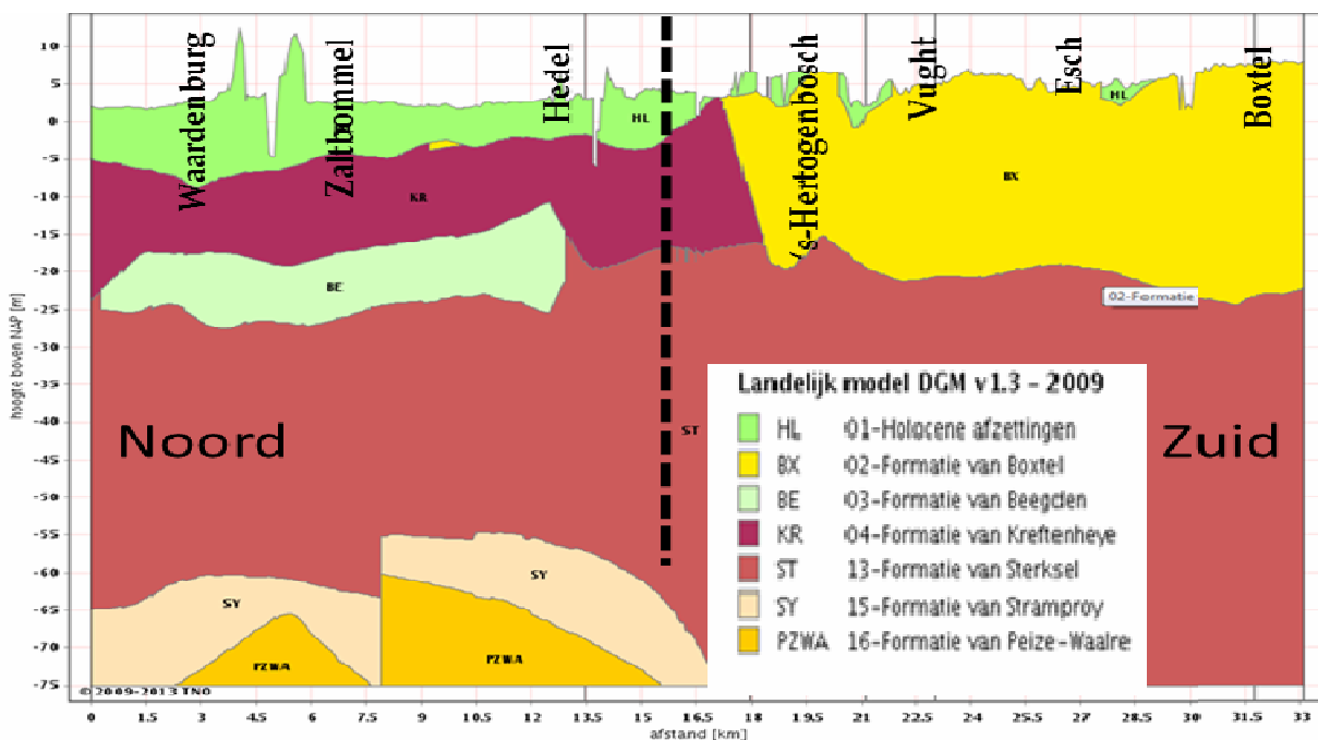
Figuur 14 Geologisch lengteprofiel ondergrond
