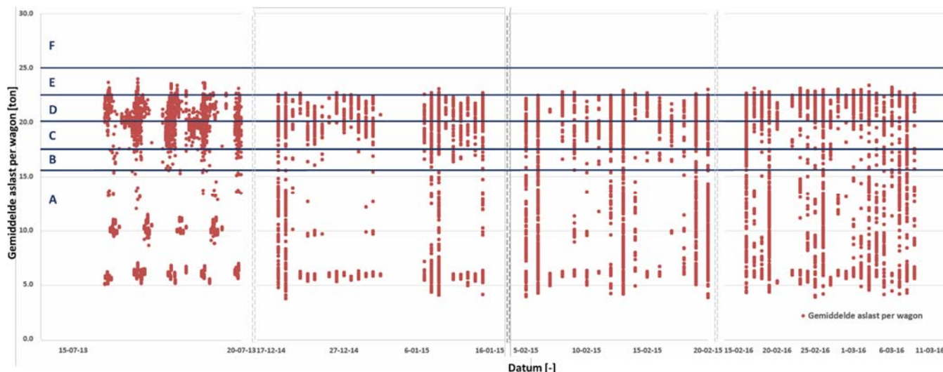
Figuur 13 Aslasten goederentreinen traject Vught - Aansluiting Vught
