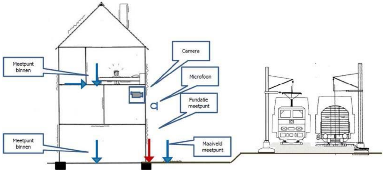
Figuur 17 Meetopstelling meting aan bebouwing
