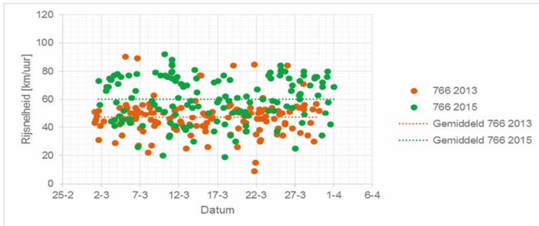
Figuur 10 Rijsnelheid goederentreinen westelijk spoor 766, gedurende maart 2013 en maart 2015
