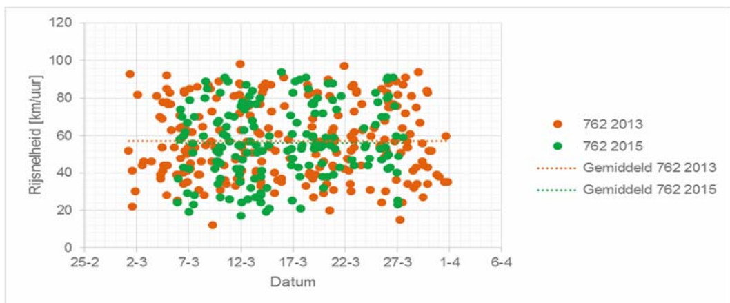
Figuur 11 Rijsnelheid goederentreinen middelste spoor 762, gedurende maart 2013 en maart 2015
