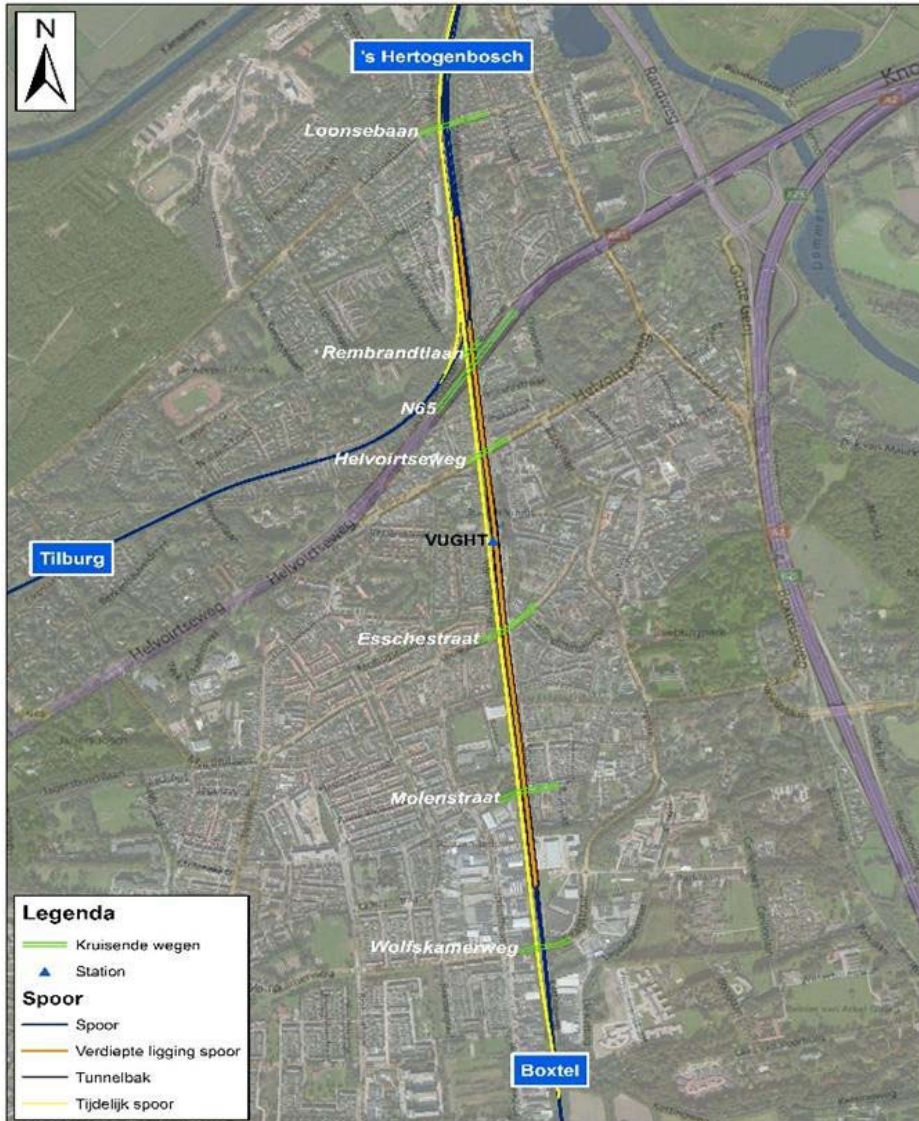
Figuur 6: Verdiepte ligging in Vught
