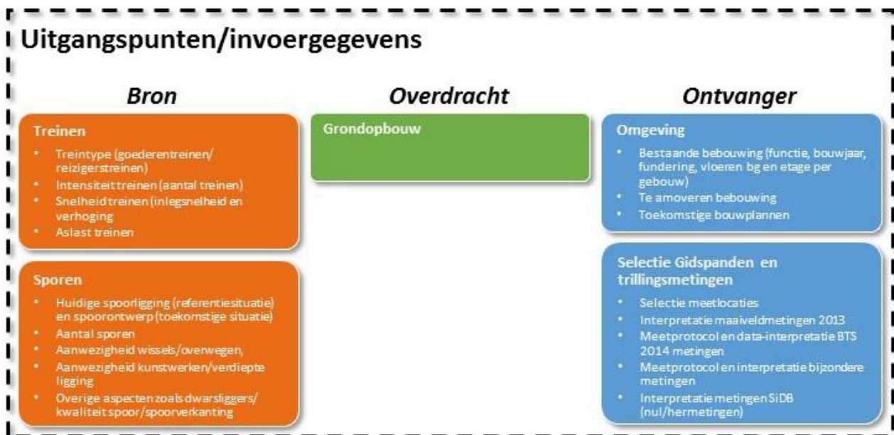
Figuur 9 Schematisch overzicht bron-, overdracht- en ontvanger gerelateerde uitgangspunten/invoergegevens
