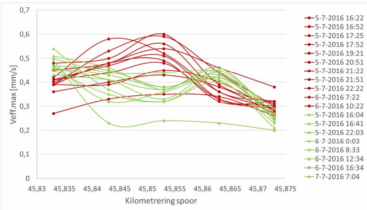
Figuur 20 Sprinters uit overweg meting Orthen (rode lijnen sprinters westelijk spoor, groene lijnen sprinters oostelijk spoor)
