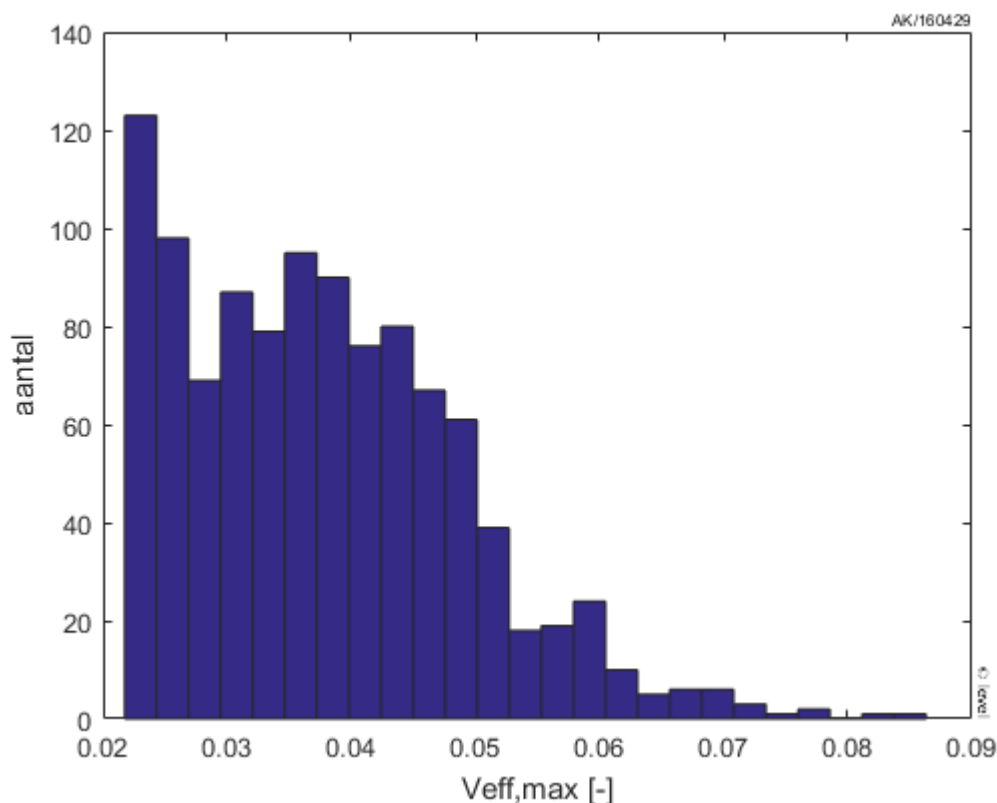
Figuur 1: TopX (1060 passages) van kanaal X van referentiepunt Majjweg (2012)
