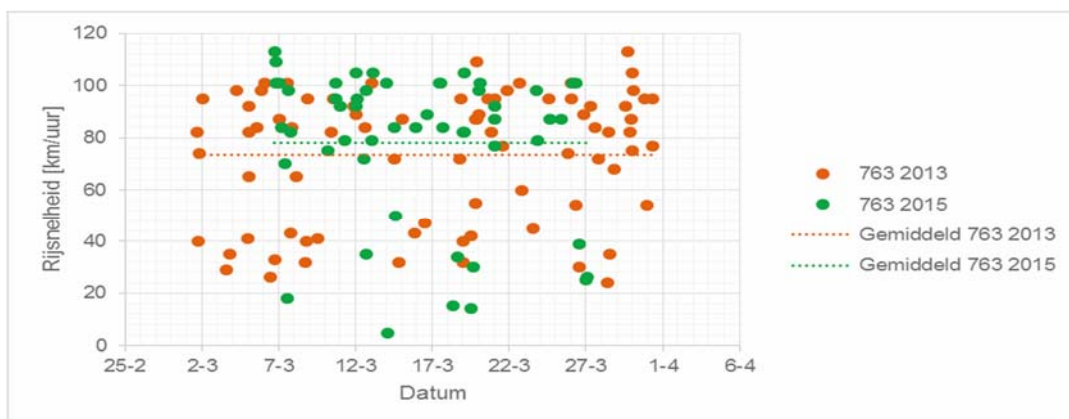
Figuur 12 Rijsnelheid goederentreinen oostelijk spoor 763, gedurende maart 2013 en maart 2015
