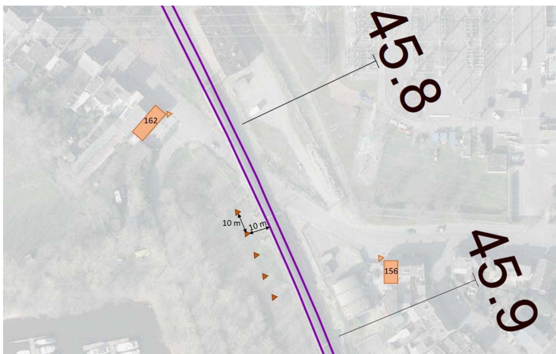
Figuur 18 Opzet trillingsmeting overweg Orthen
