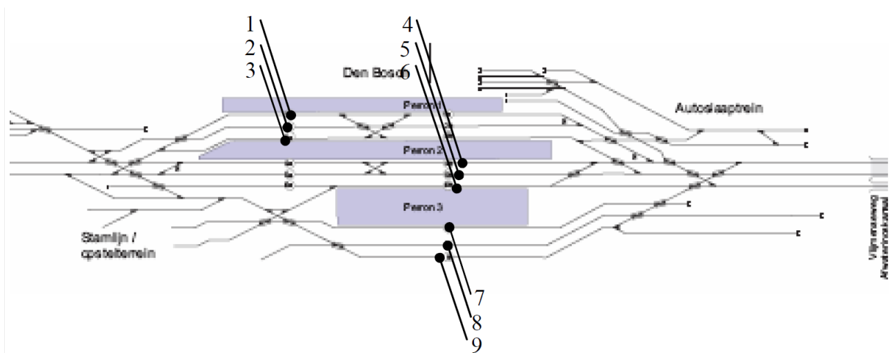
Figuur 5 Spoorligging referentiesituatie, met aangehouden nummering uit Tracébesluit Sporen in Den Bosch
