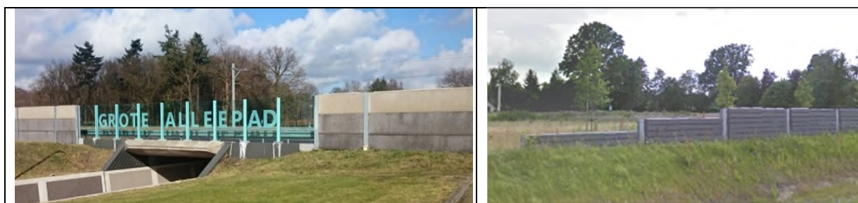
Figuur 7.4: Geluidwering type Combiplan, met rechts de getrapte opbouw
