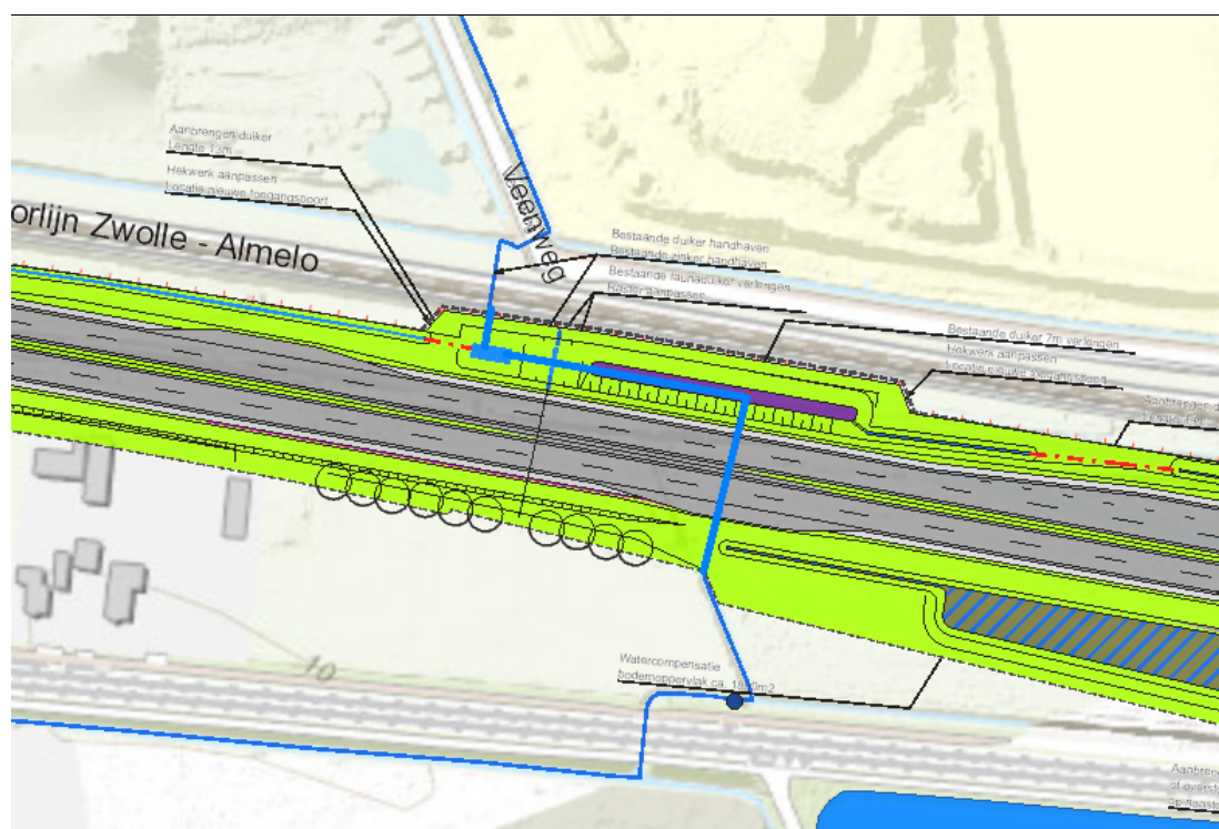
Figuur 5.2 Kruising van watergang met de N35 ter hoogte van de Veerweg (huidige situatie).
