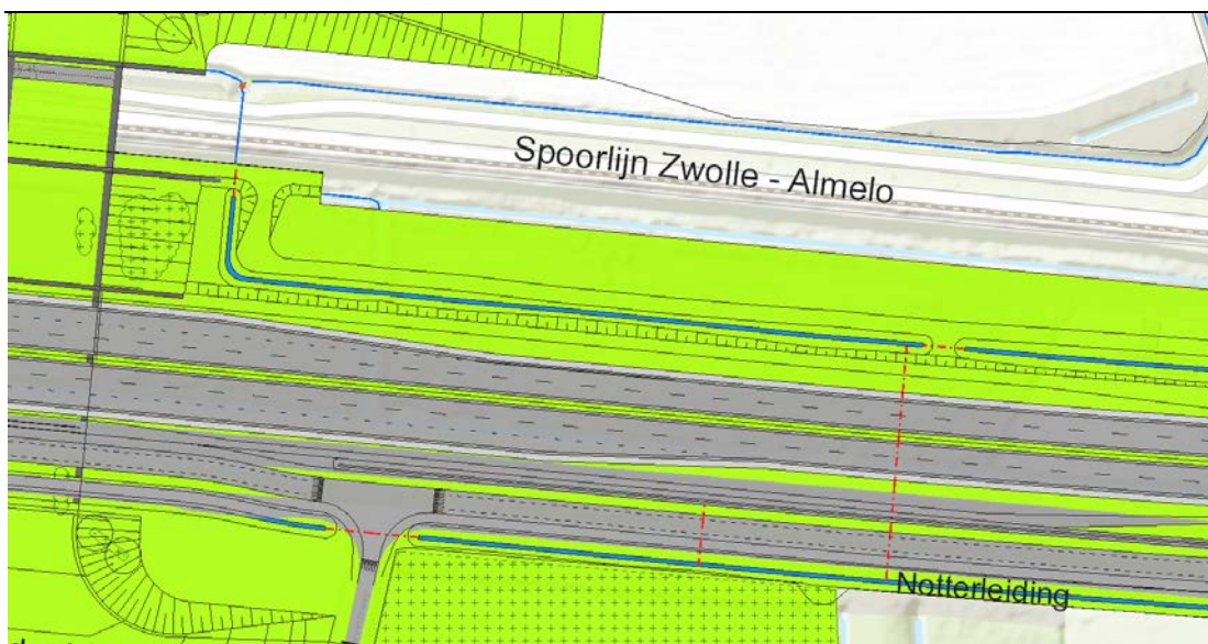
Figuur B2.3 Toekomstige situatie bij gemaal Westerveenweg met watergangen voor afvoer van water vanaf het gemaal
