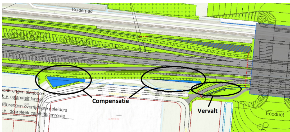
Figuur B2.1 Aanpassingen aan retentievijver aan noordkant 't Lochter III
