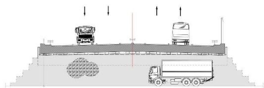
aanzicht A-A'
