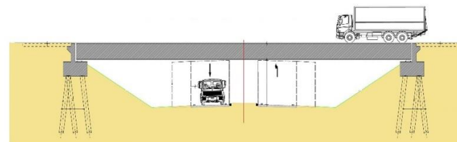
aanzicht B-B'
