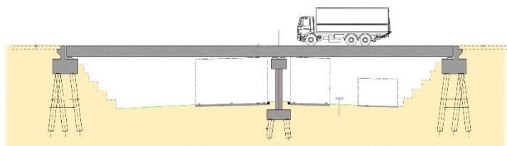
langsdoorsnede B-B'
