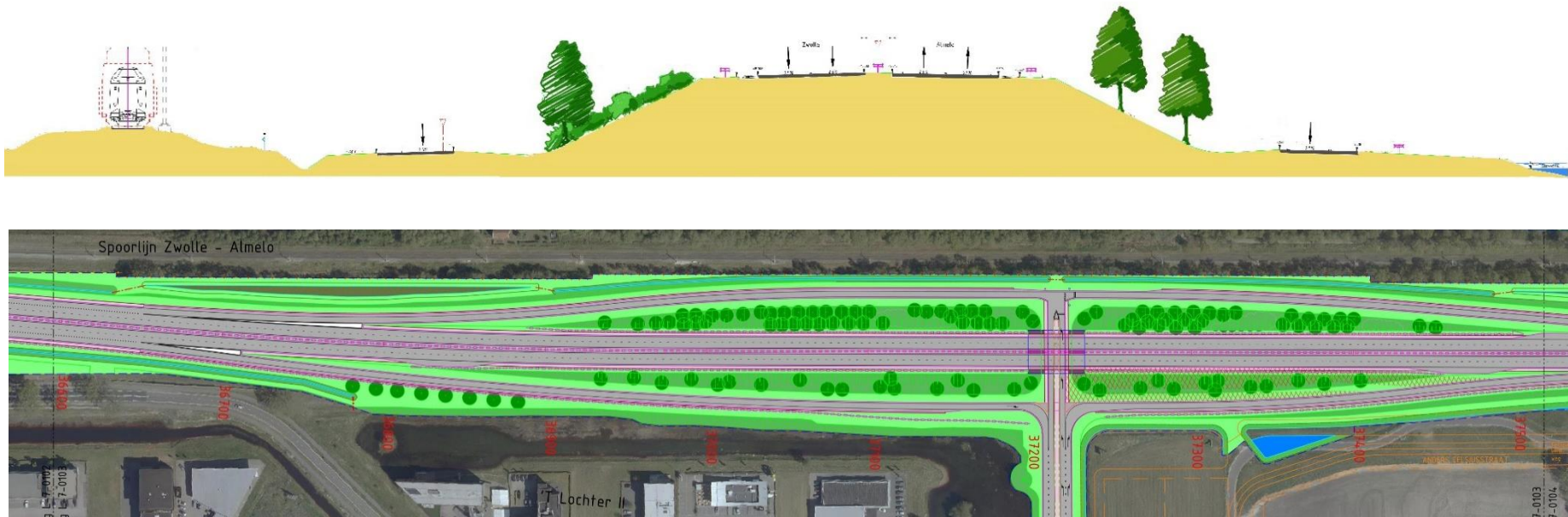
Figuur 6.8 Natuurlijke beplanting aan de noordzijde en parkachtige beplanting aan de zuidzijde van de aansluiting Burg. H. Boersingel
