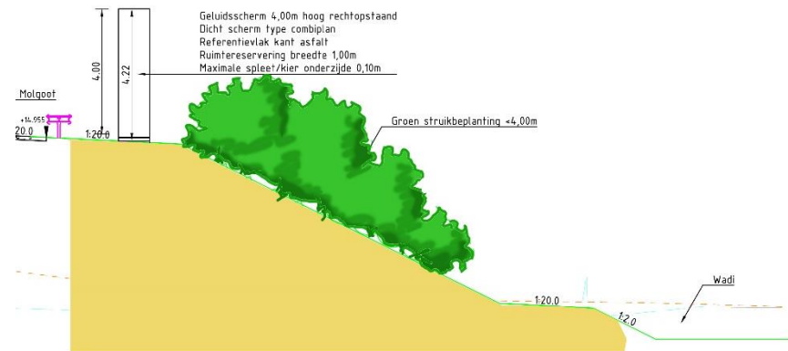
Figuur 6.16 Beplanting achter het geluidsscherm mag niet boven het scherm uitgroeien om verstrooiing en reflectie van het geluid tegen te gaan
