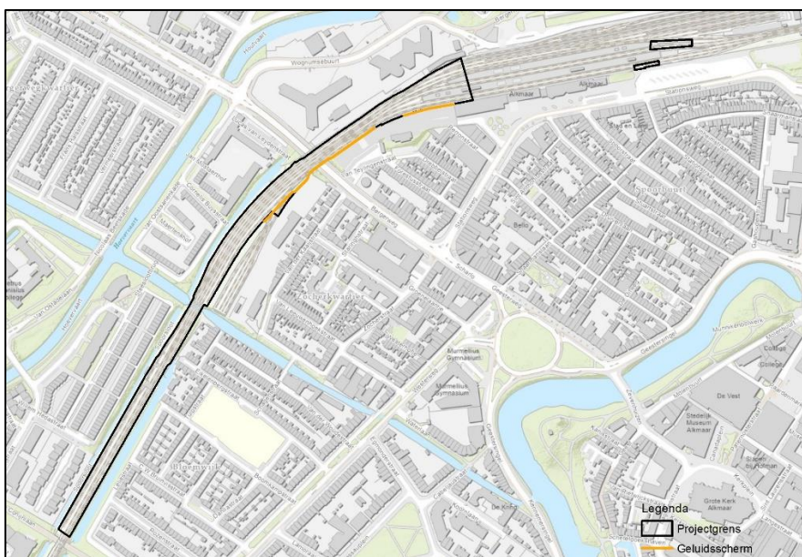
Figuur 2 Projectgebied PHS Alkmaar-Amsterdam: Station Alkmaar
