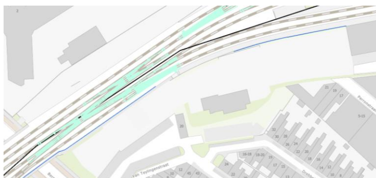
Figuur 4.22 Locatie geluisschermen emplacement Alkmaar
