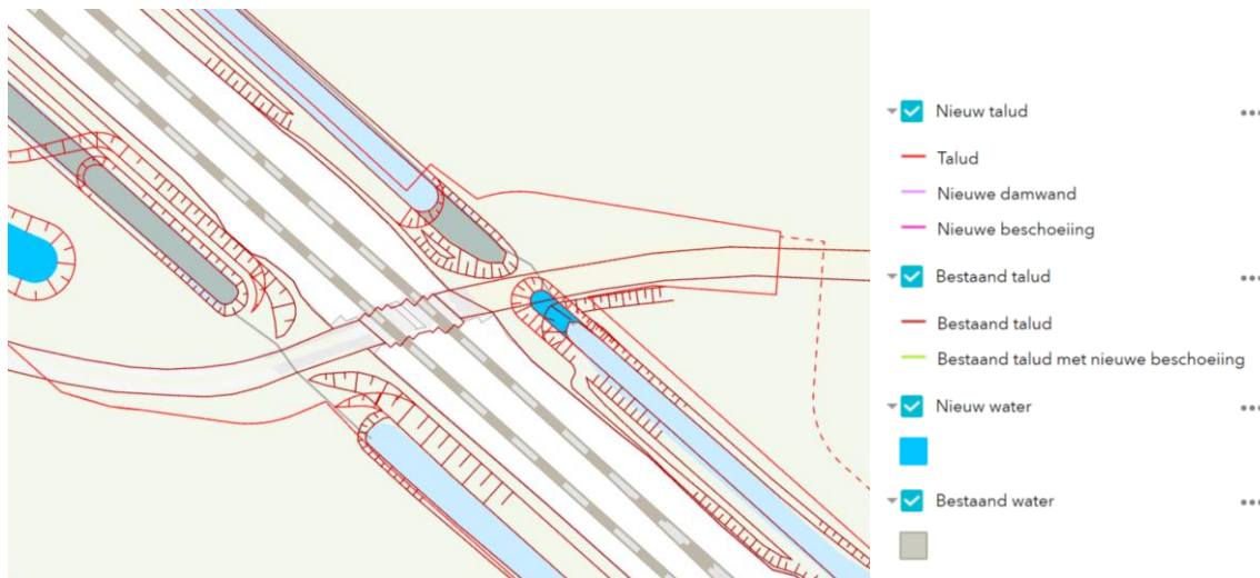
Figuur 4.8 Detail spoorwegovergang ten westen van Uitgeest
