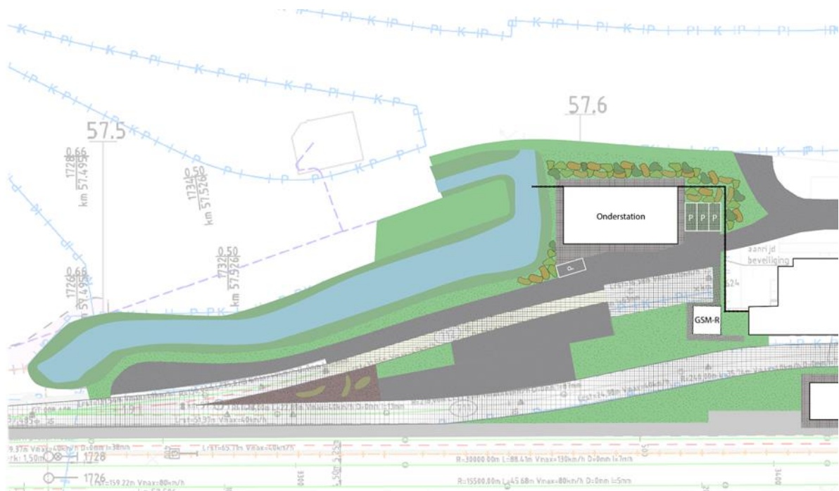
Figuur 4.19 Inpassingsplan terrein ten noordwesten van station Uitgeest met hierop het onderstation (boven) en de GSM-mast.
