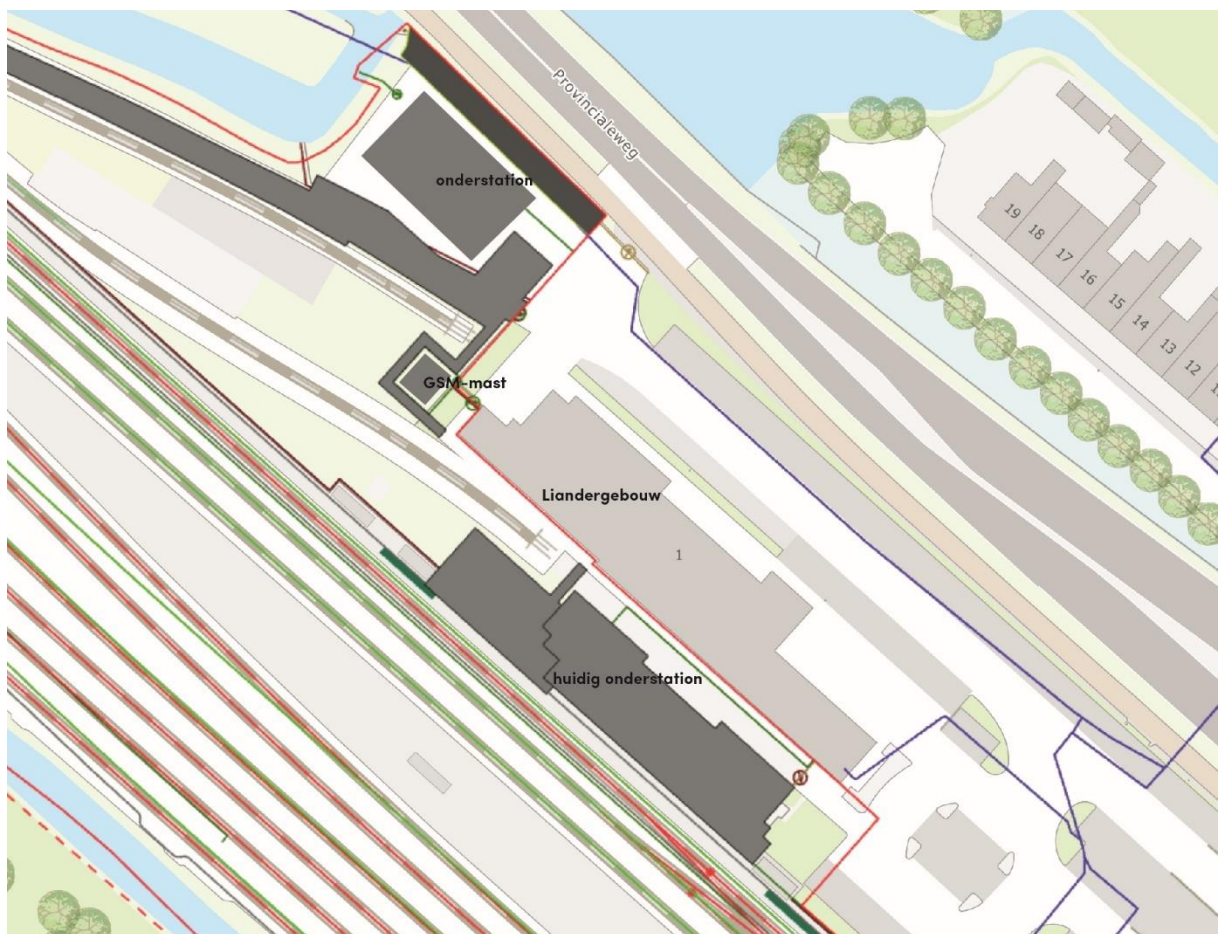
Figuur 4.11 Locatie en plaatsing onderstation en relaishuis
