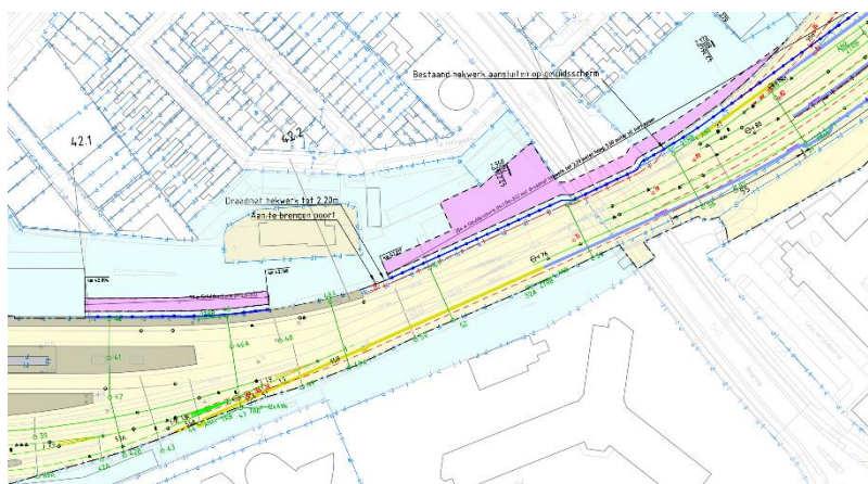
Figuur 4.23 Situatie spoorwegviaduct Bergerweg
