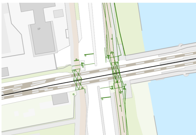
Figuur 4.20 Ontwerptekening overweg Helderseweg
