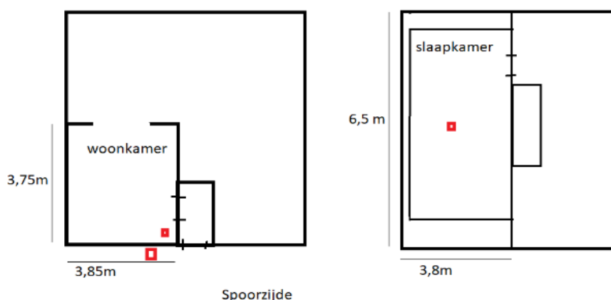
Figuur 3.3: Schets plattegrond met meetposities Parallelweg 27. Alleen ruimtes waarin is gemeten zijn afgebeeld. De rode vierkanten geven de meetposities weer.
