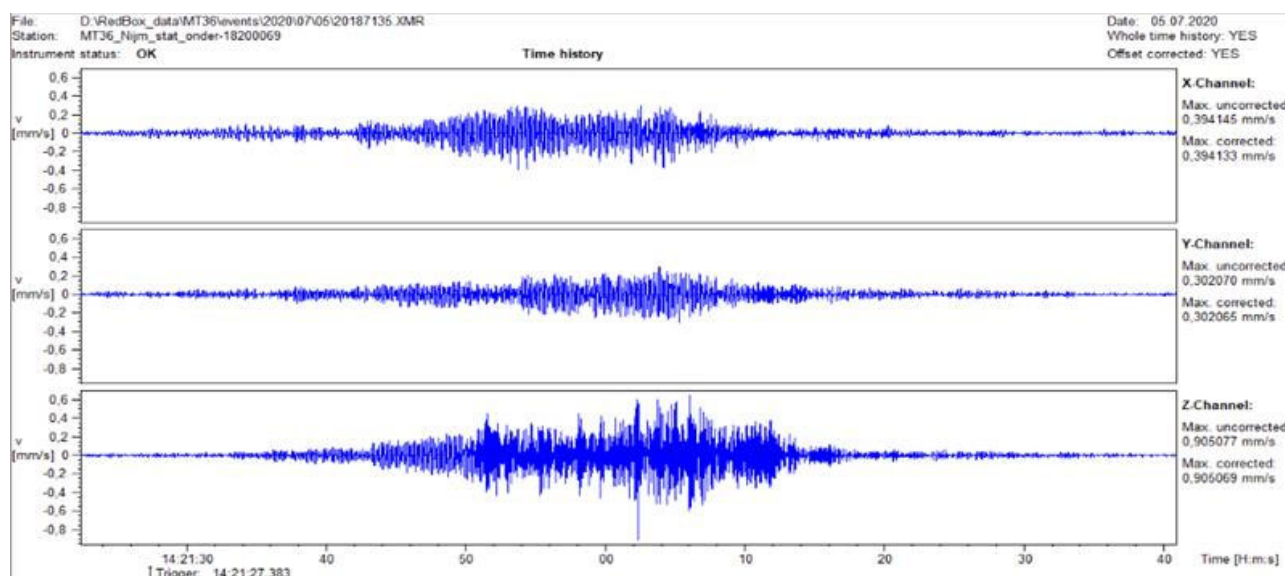
Figuur 4.1: Tijdsignaal passage trein V_{top} Stationsweg
