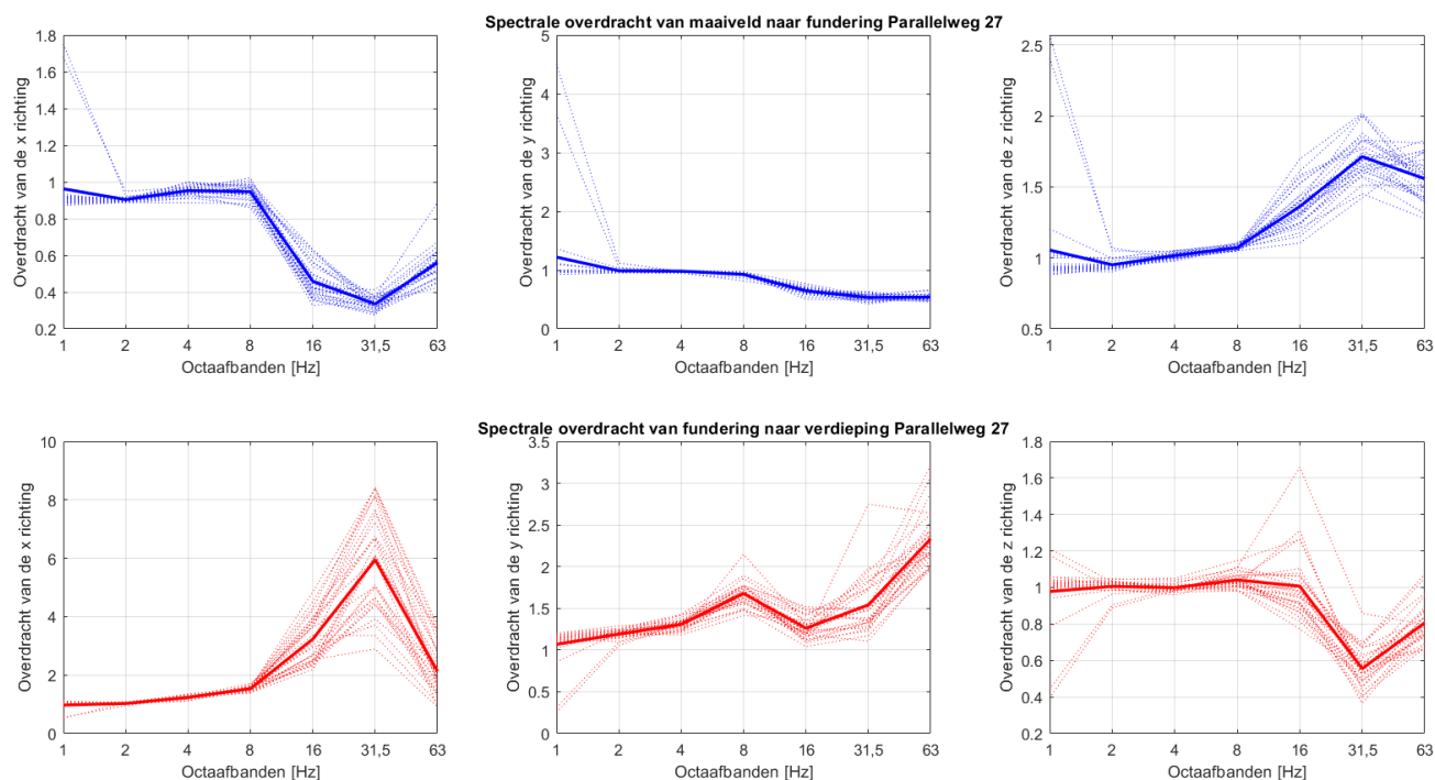
Figuur 4.2: Spectrale overdracht Parallelweg 27
