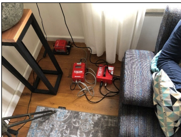
Figuur 3.12: Meetpunt fundering (MT36) in de hoek van de woning op de begane grond
