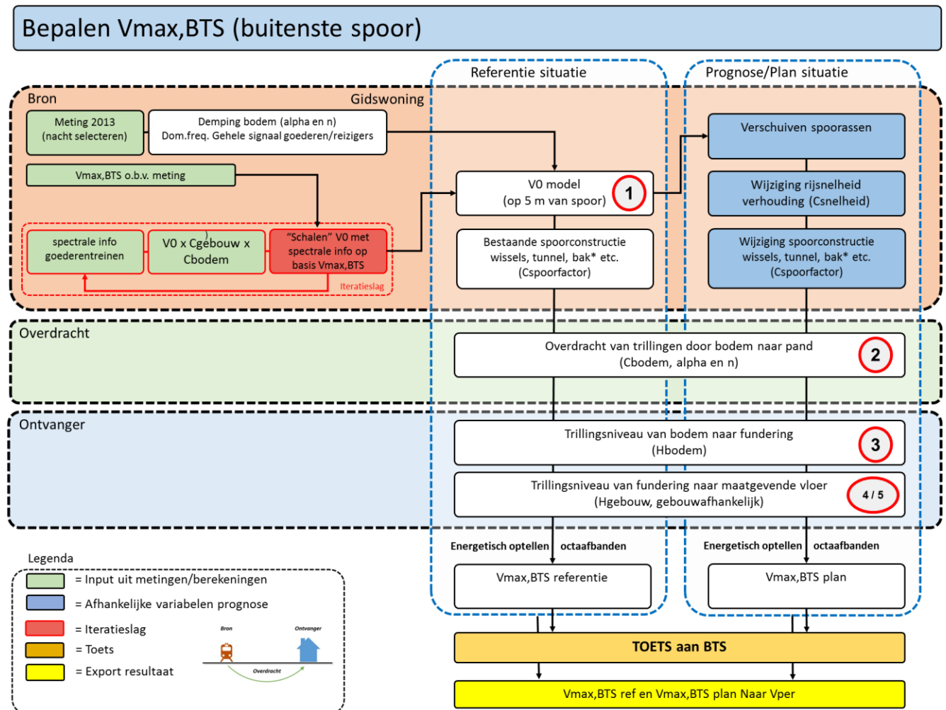
Figuur 9 Stroomschema V_{max}
