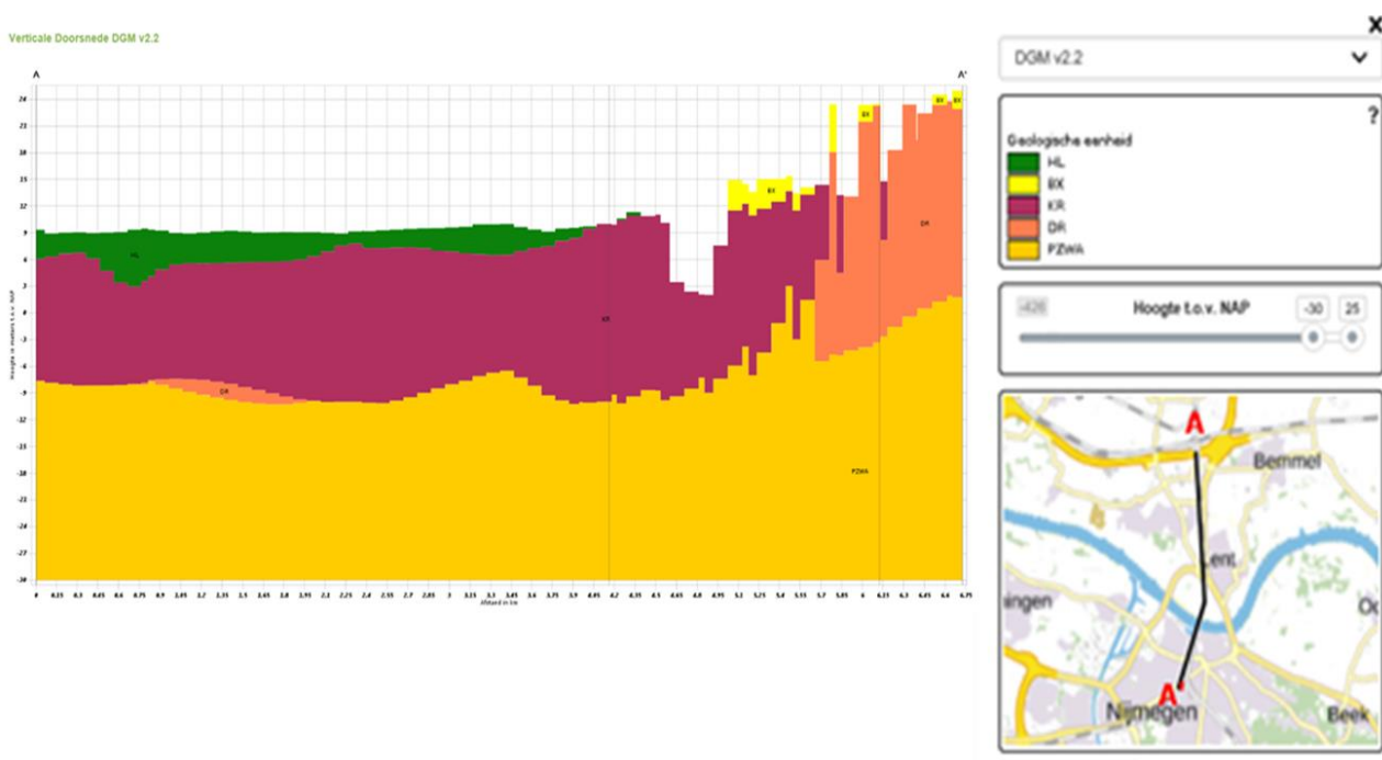
Figuur 7: Geologisch langsprofiel spoorlijn Arnhem- Nijmegen (bron: DGM versie 2.2, Dino Loket)
