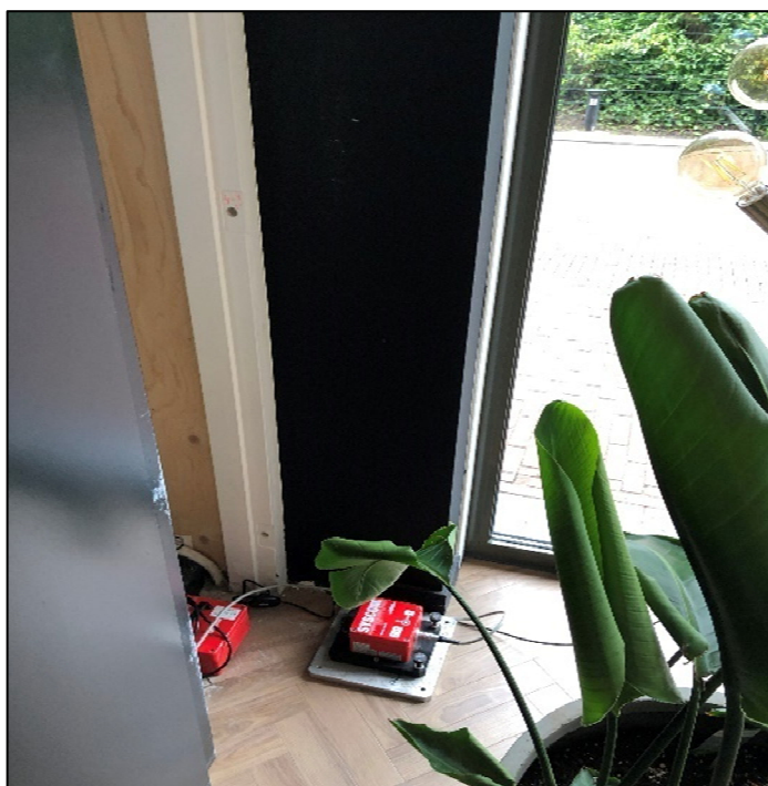
Figuur 3.17: Meetpunt fundering (ZT47) Dokstraat
