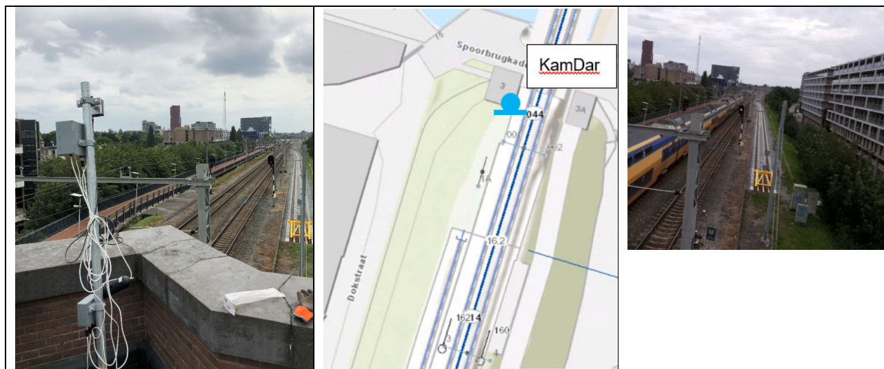
Figuur 3.21: KamDar op het Landhoofd Dokstraat (links) en beeld van de KamDar (rechts)
