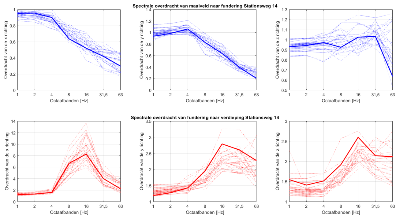
Figuur 4.3: Spectrale overdrachten woning Stationsweg 14
