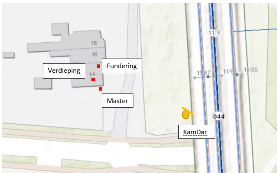
Figuur 3.10: Bovenaanzicht woning en spoor. Rode vierkanten zijn de meetpunten en de gele bol is de Kamdar
