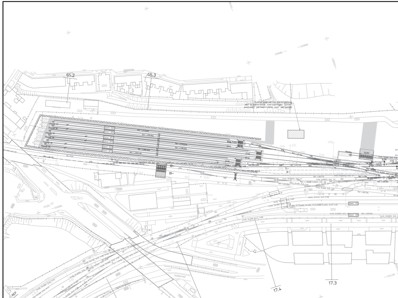
Technisch spoorontwerp zuidzijde (concept 10-04-2020)
