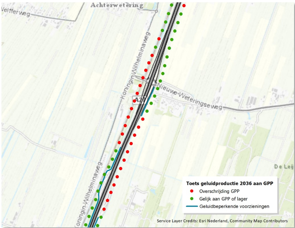
Figuur 24 – Overschrijdingen GPP's bij Nieuwe Wetering
