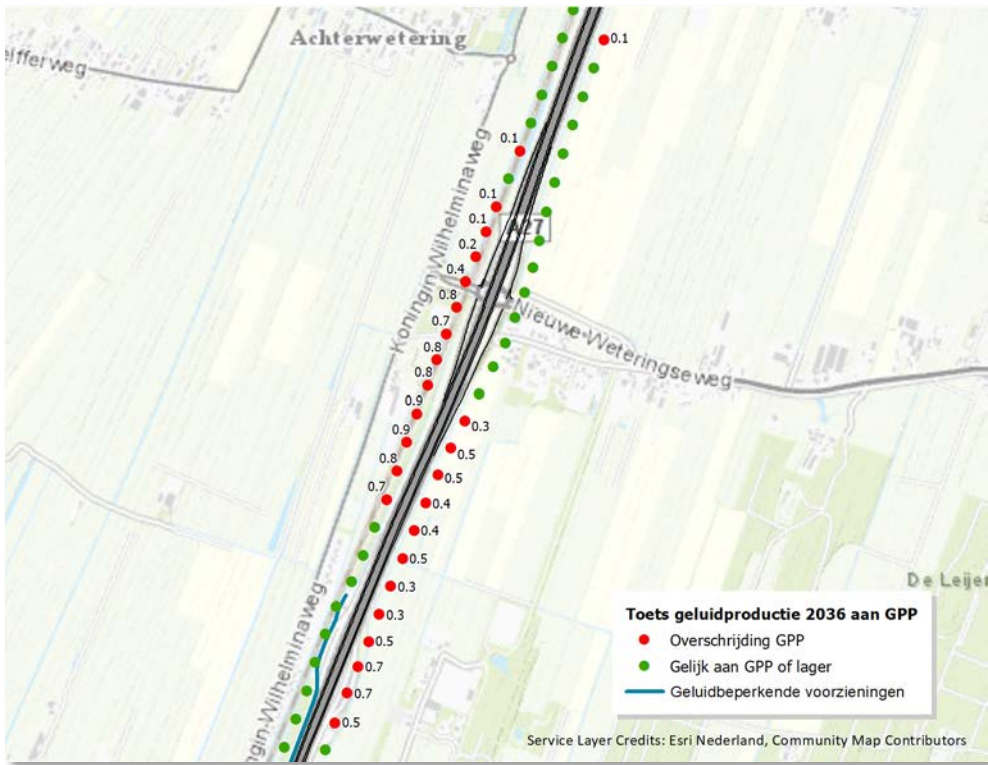
Figuur 19 – Overschrijdingen GPP's bij Nieuwe Wetering
