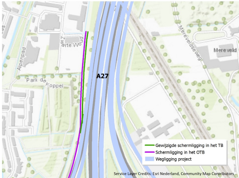
Figuur 2 Gewijzigde schermligging verbindingsweg A27 naar A12 bij Lunetten
