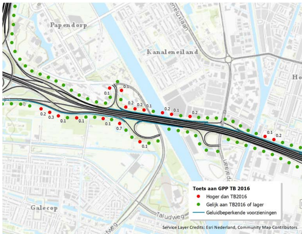
Figuur 18 – GPP's bij TB2020 hoger dan bij TB2016 bij Nieuwegein en Kanaleneiland
