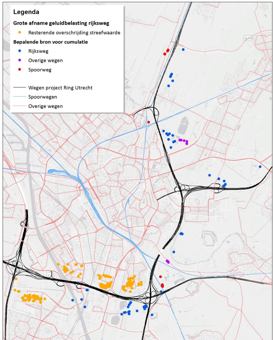
Figuur 32 Resterende overschrijdingen met categorie cumulatieve situatie
