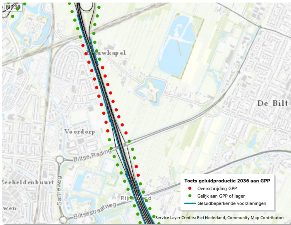
Figuur 25 – Overschrijdingen GPP's ter hoogte van Voordorp
