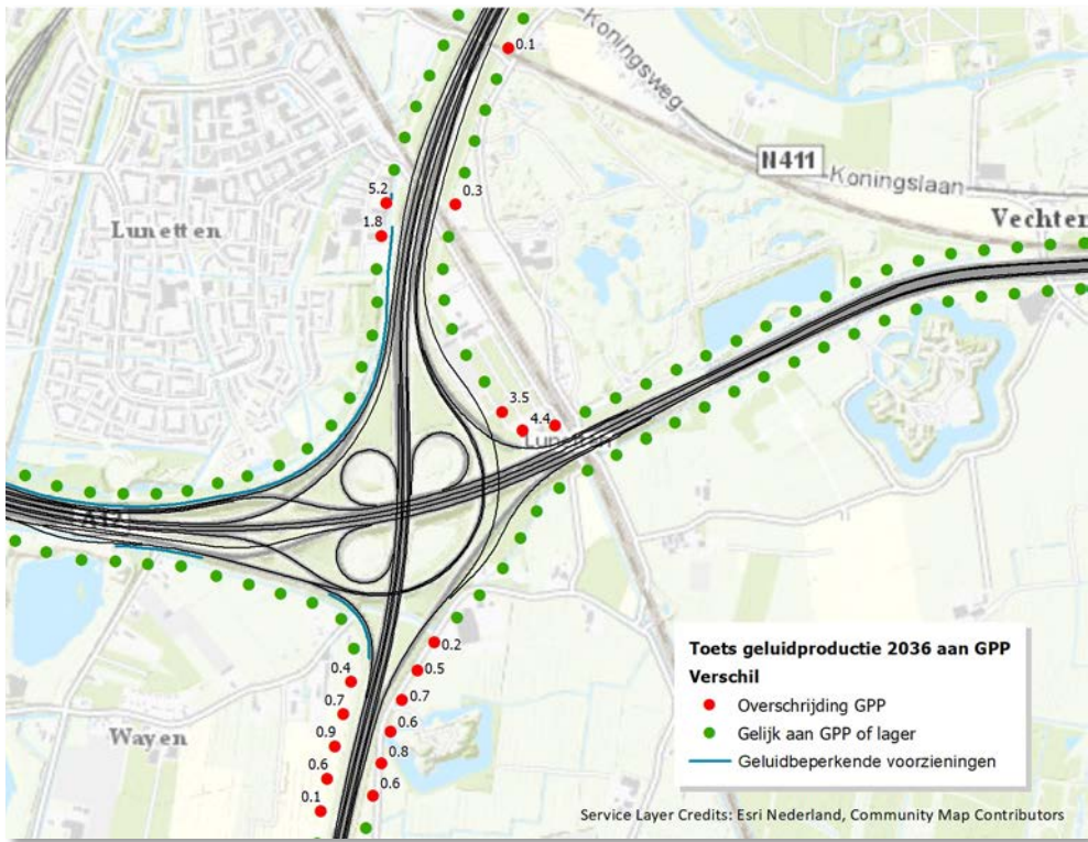
Figuur 23 – Overschrijdingen GPP's rond knooppunt Lunetten
