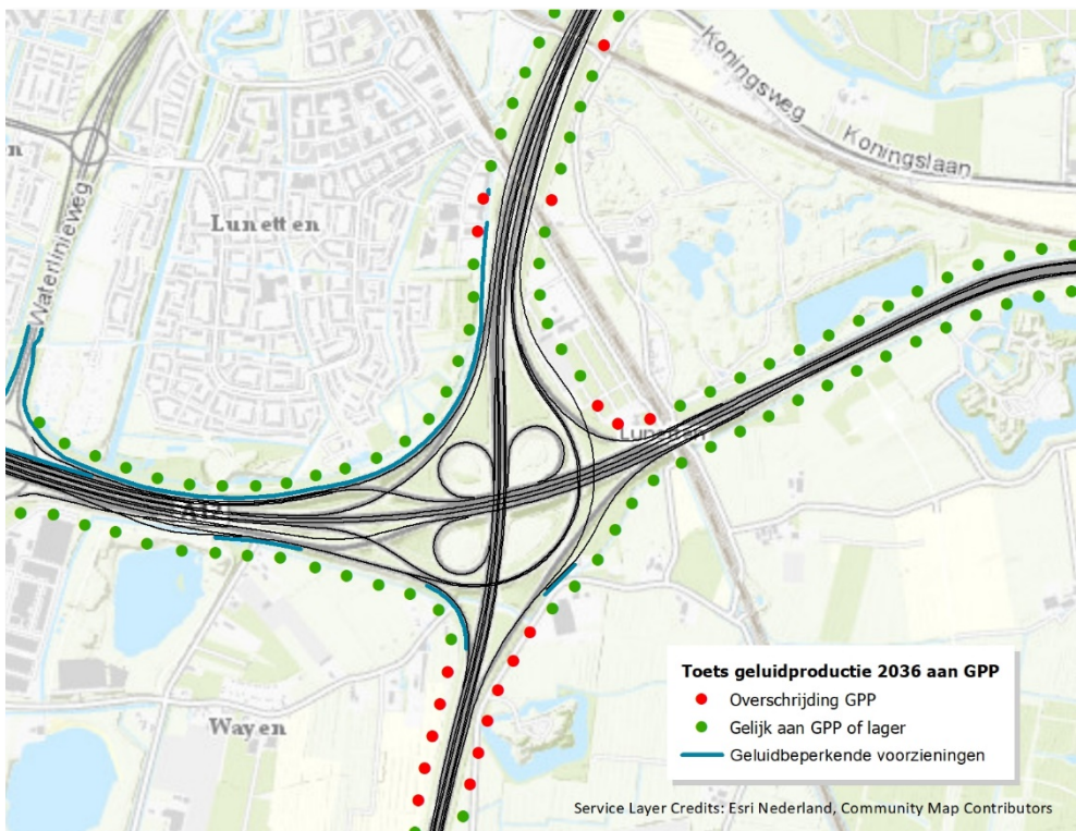
Figuur 28 – Overschrijdingen GPP's ter hoogte van knooppunt Lunetten
