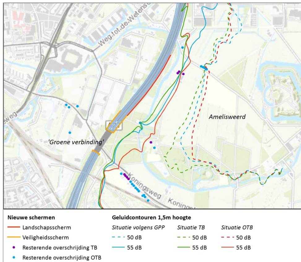
Figuur 10 Geluidcontouren en resterende overschrijdingen rond bak Amelisweerd
