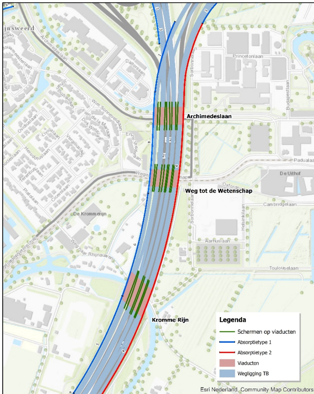
Figuur 7 Overzicht aanvullende schermen viaducten
