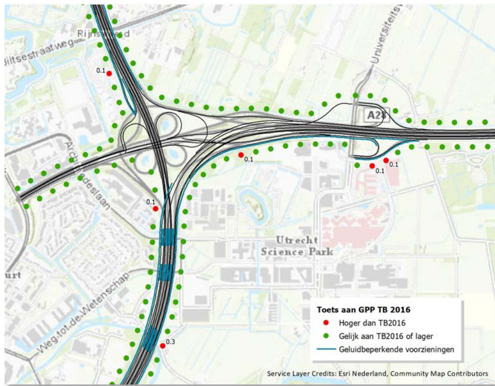
Figuur 16 – GPP's bij TB2020 hoger dan bij TB2016, omgeving Rijnsweerd
