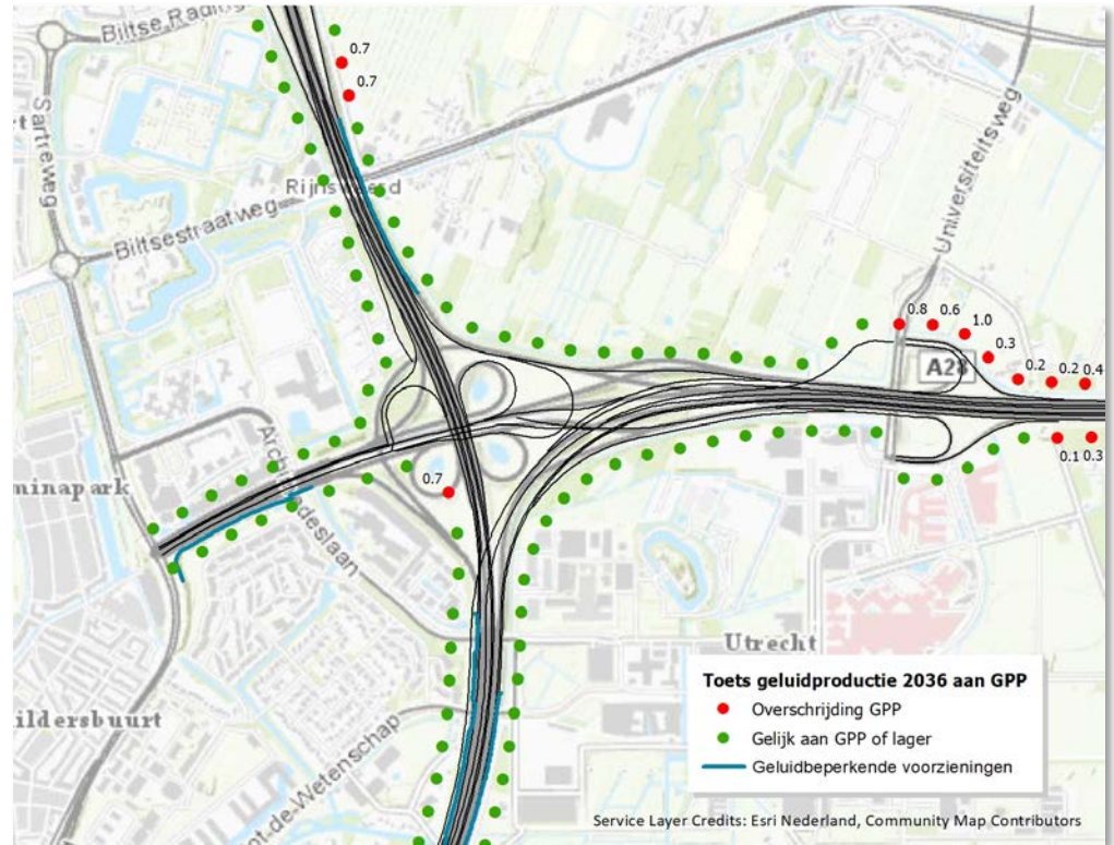
Figuur 21 – Overschrijdingen GPP's rond knooppunt Rijnsweerd
