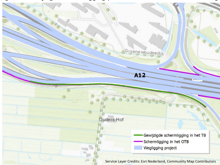
Figuur 1 Gewijzigde schermligging parallelbaan A12 naar afrit Nieuwegein
