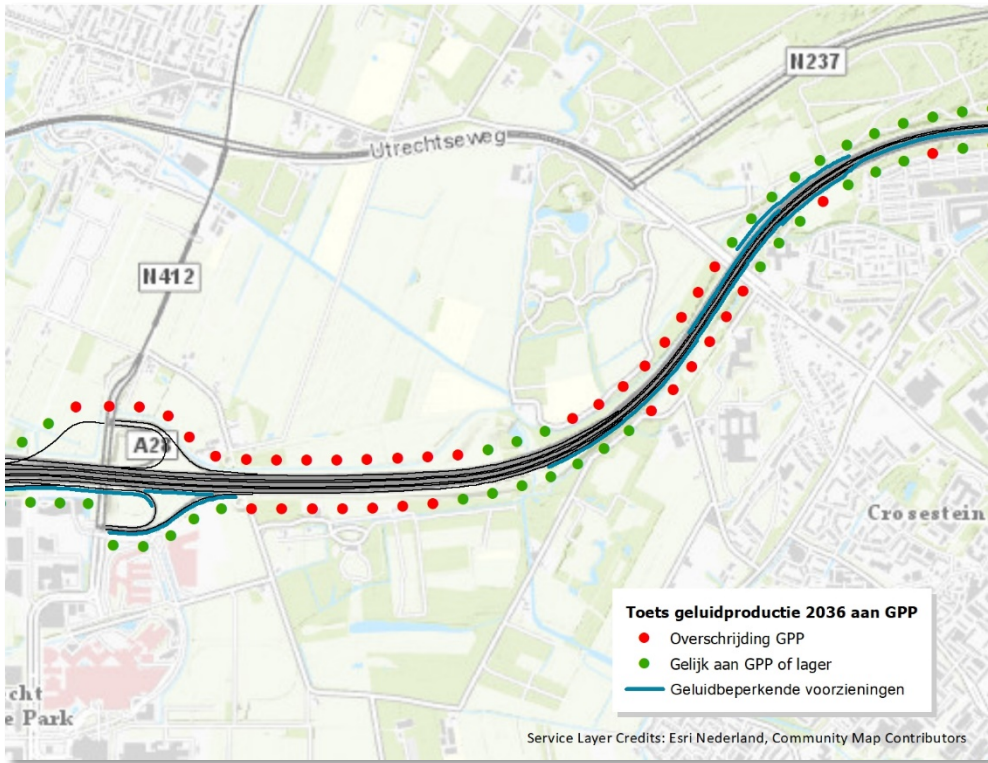
Figuur 27 – Overschrijdingen GPP's tussen de aansluiting de Uithof en Zeist
