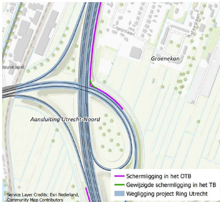
Figuur 4 Gewijzigde schermlijging zuidzijde Groenekan
