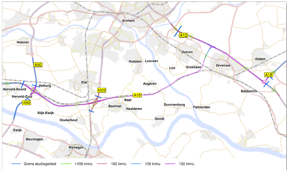
Figuur 7 Globaal overzicht maximumsnelheden die als uitgangspunt zijn gehanteerd in de geluidberekeningen
