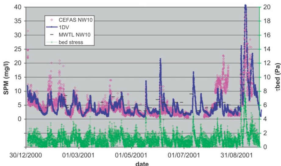
Figuur B.2 Vergelijking tussen een 1Dv slibmodel (paarse lijn) en hoogfrequente slibmetingen (wiebertjes) respectievelijk MWTN-metingen (streepjes) in 2001 voor het station Noordwijk 10 (Van Kessel et al., 2011).
