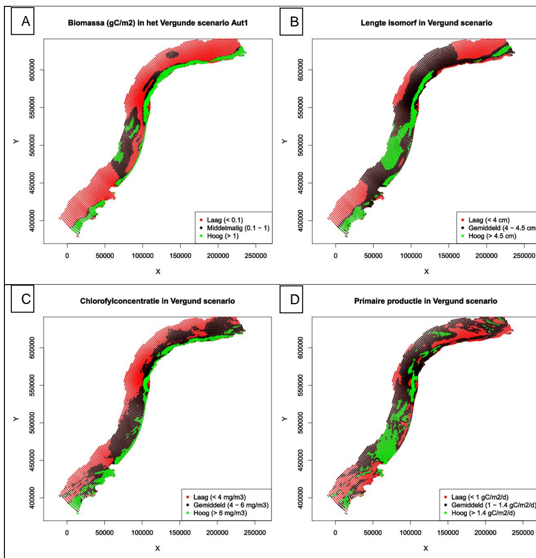
Figuur 7.2 Ruimtelijke verdeling van a) biomassa van de V1 morf van Ensis (gC/m 2 ); b) lengte van de juveniele isomorf op 1 december (cm); c) chlorofylconcentratie in de onderste waterlaag (mg/m 3 ) d) primaire productie geïntegreerd over de waterkolom (gC/m 2 /d). Alle gegevens zijn voor het Vergunde scenario in 2027. Behalve voor de lengte van de isomorf betreft het jaargemiddelden.
