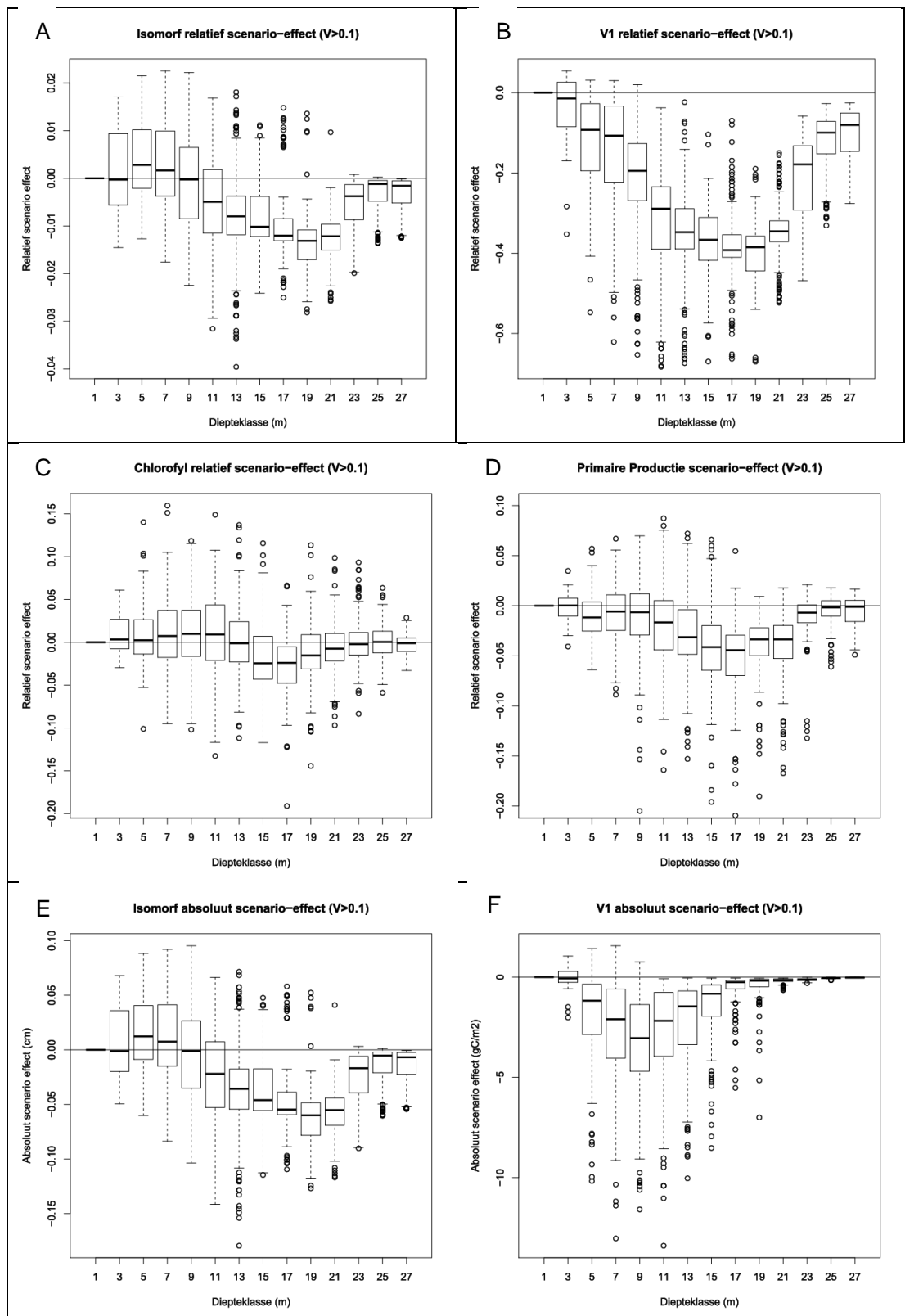
Figuur 7.5 Scenario-effect van het cumulatieve scenario ten opzichte van het vergunde scenario. a) relatief effect op de lengte van isomorfen; b) relatief effect op de biomassa van de V1; c) relatief effect op chlorofyl; d) relatief effect op primaire productie; e) absoluut effect op de lengte van de isomorfen; e) absoluut effect op de biomassa van de V1. Alle berekeningen gebaseerd op het jaar 2027
