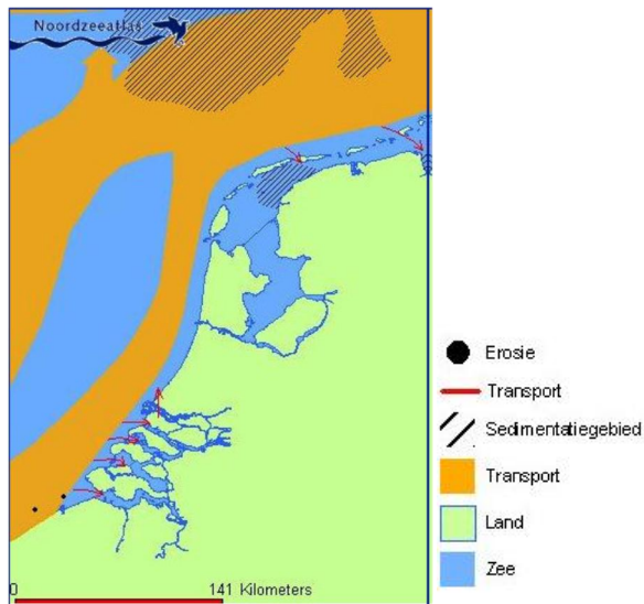
Figuur 2.3 Slibtransport in de Noordzee
