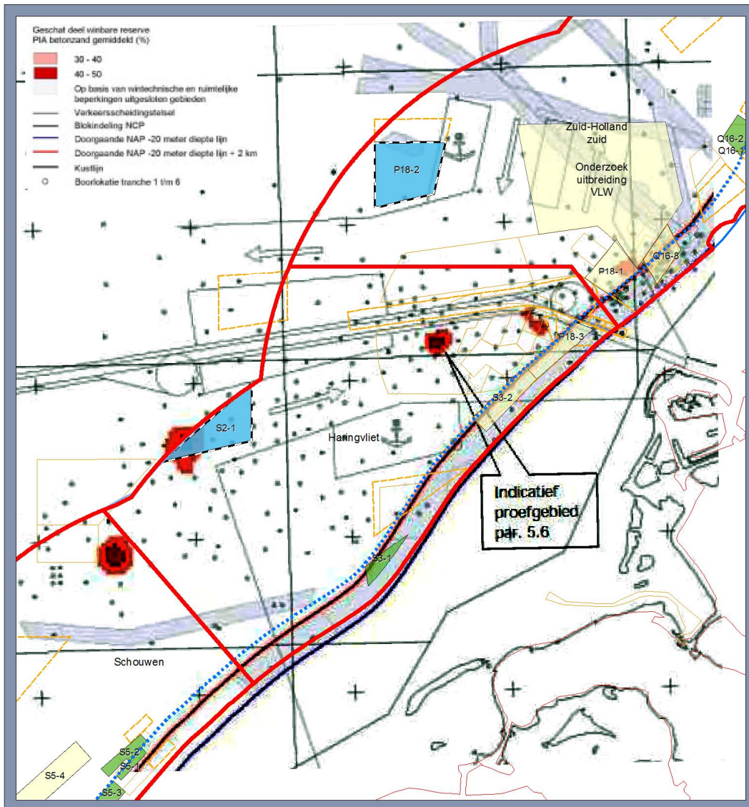
Figuur 12.9 Ligging zoekgebieden ten opzichte van de kansrijke voorkomens van beton- en metselzand
